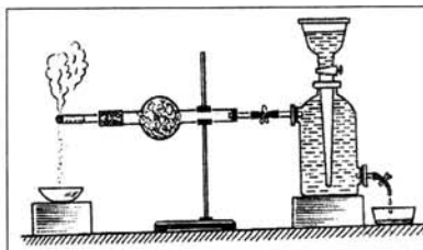
Рисунок № 1. Установка для демонстрации опыта «Курильщик»
